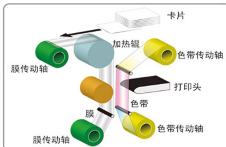
FA-P9600 打印原理示意图
